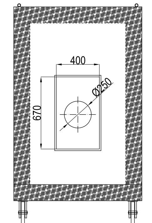
SEZ. AA
