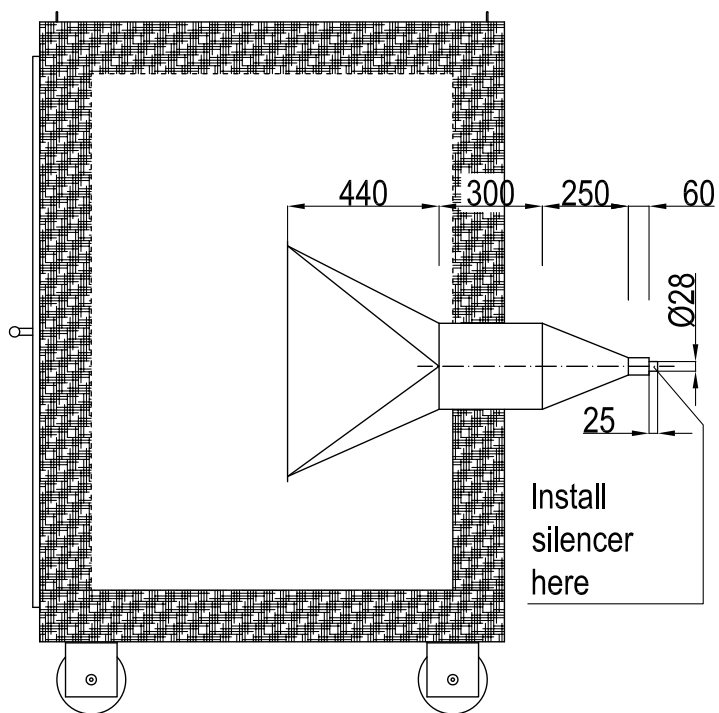
SEZ. BB
