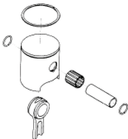
Dessin / Drawing 8.4a: Eléments considérés pour la masse alternative Elements considered for the alternative mass
