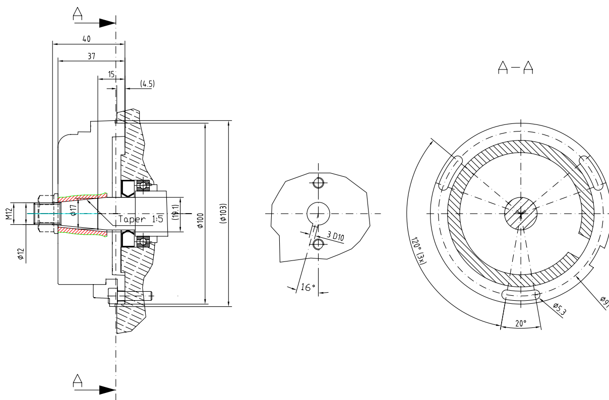
Dessin 8.5 : Schéma de principe avec dimensions obligatoires pour la fixation du rotor et du stator des allumages homologués en OK et OK-Junior
