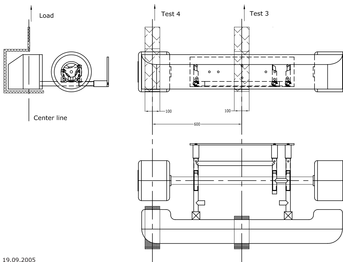
Dessin / Drawing 8.4a: Eléments considérés pour la masse alternative Elements considered for the alternative mass
