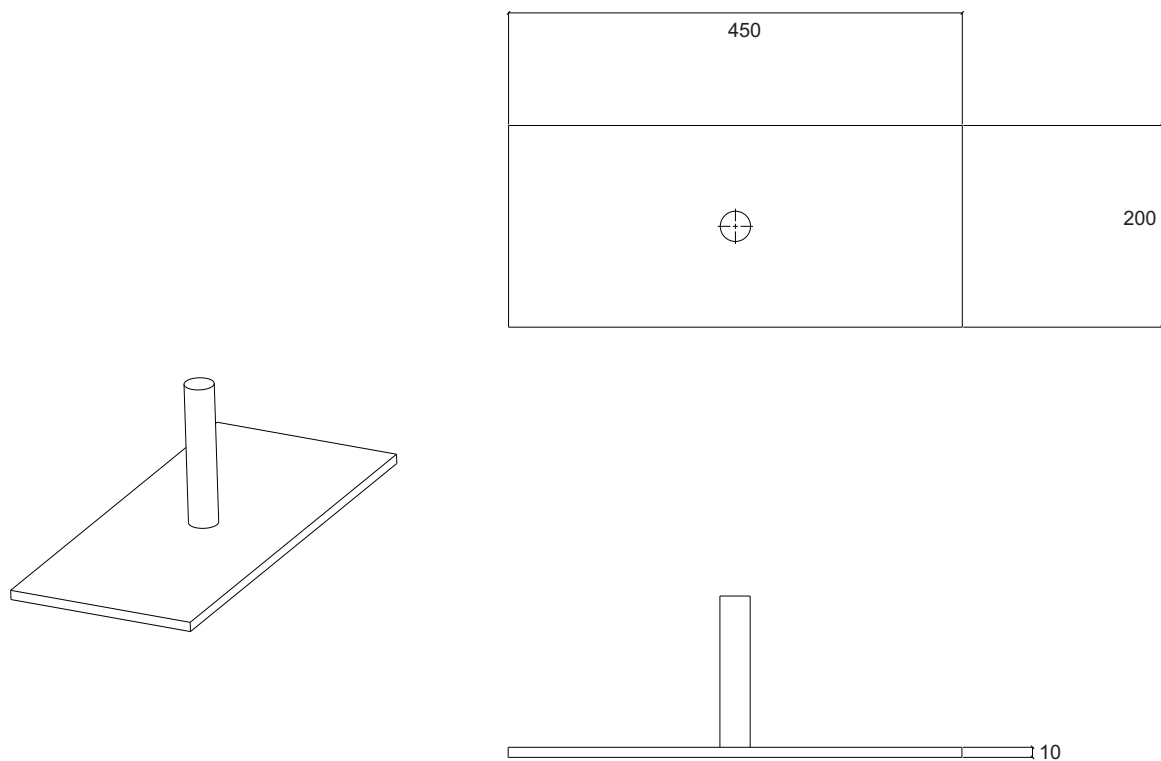
Dessin 8.2.0.a : Plaque pour essais de poussée verticale Carénage avant
