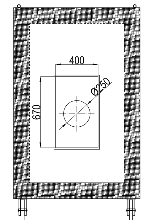
SEZ. AA
