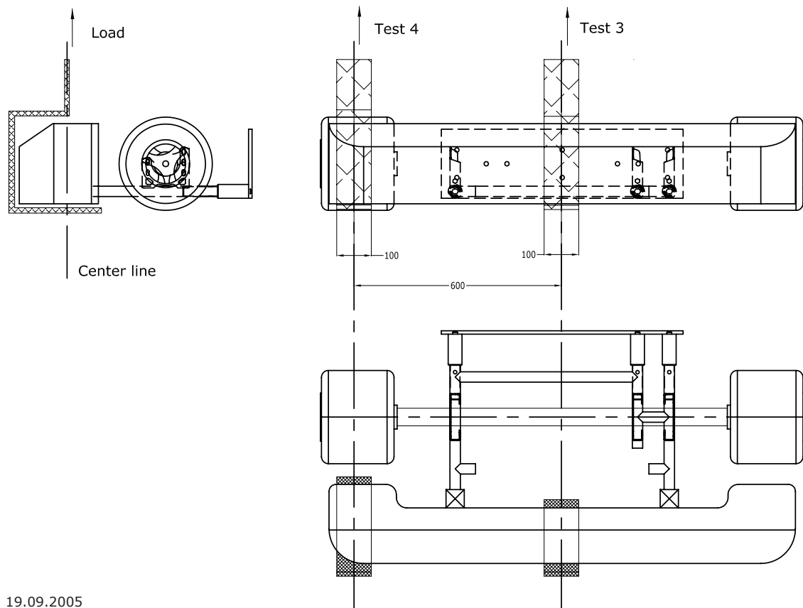
Dessin / Drawing 8.4a: Eléments considérés pour la masse alternative Elements considered for the alternative mass
