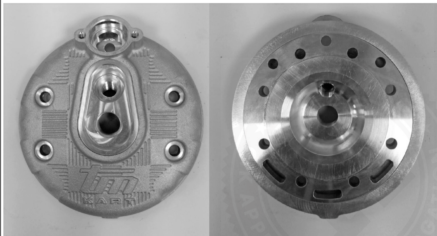
Photo de la culasse et de la chambre de combustion / Photo of the cylinder head and the combustion chamber
